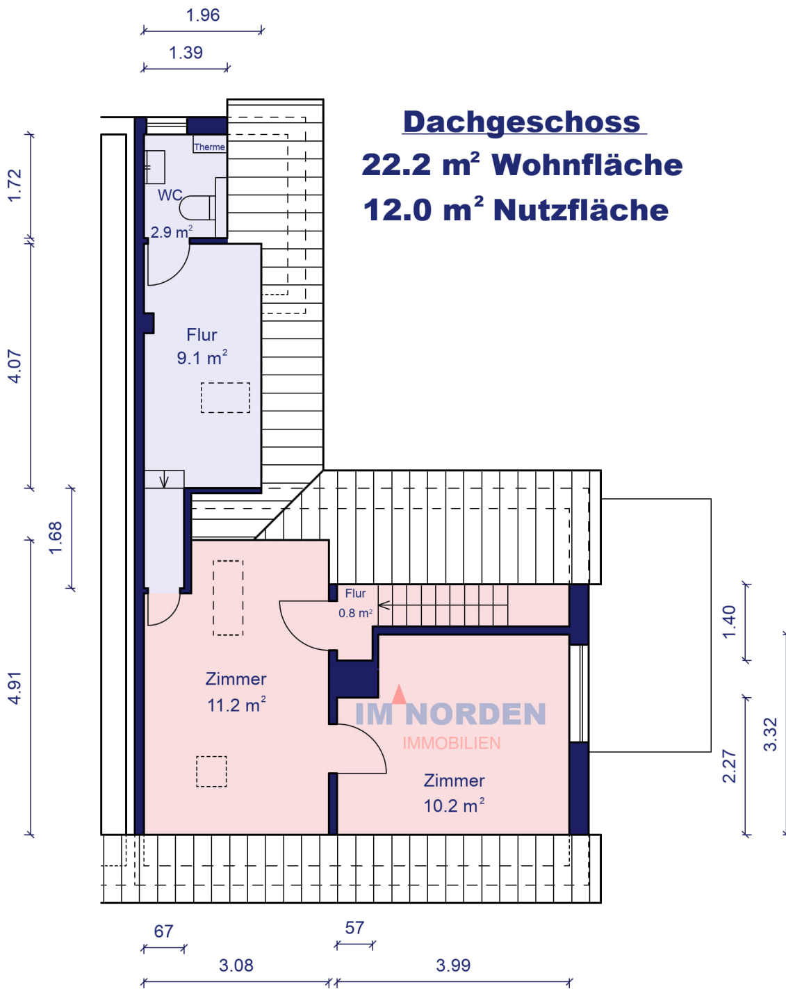
Grundriss Dachgeschoss
