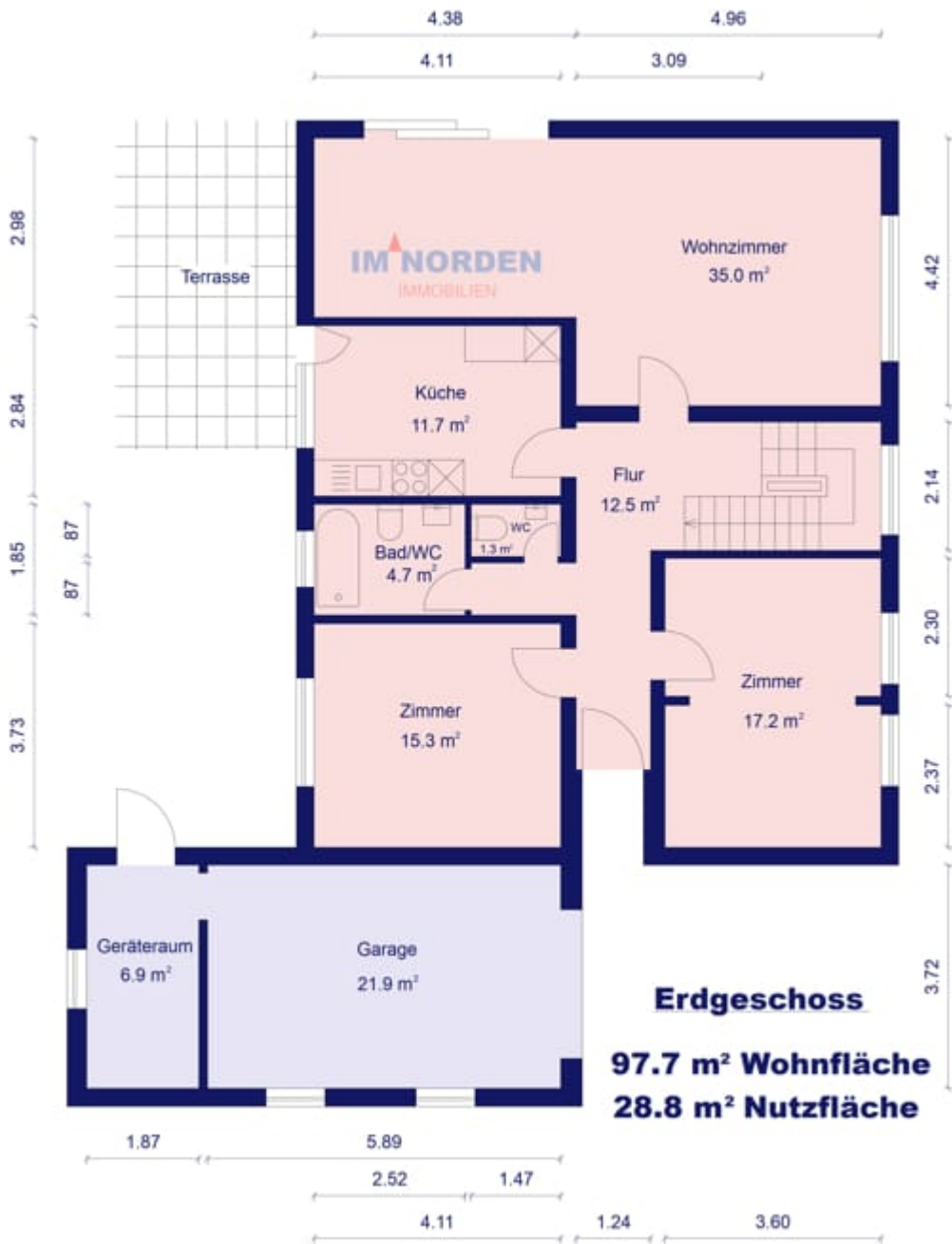
Grundriss Erdgeschoss
