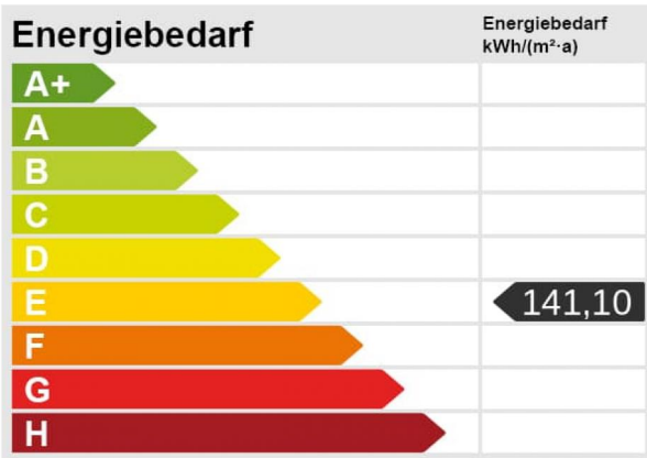
Energieskala
