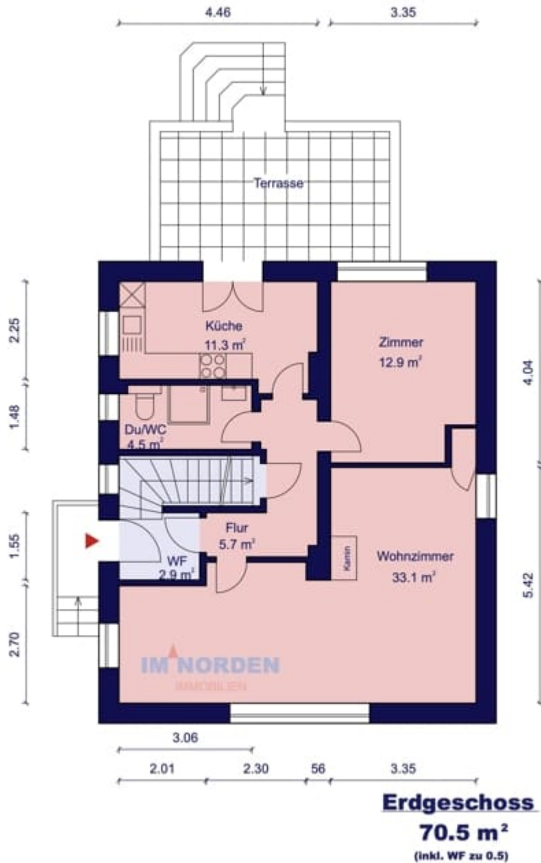
Grundriss Erdgeschoss
