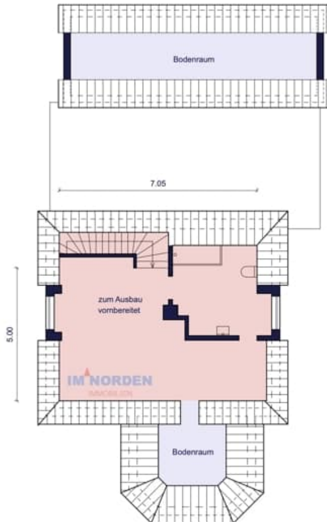
Dachgeschoss rd. 30 m 2
