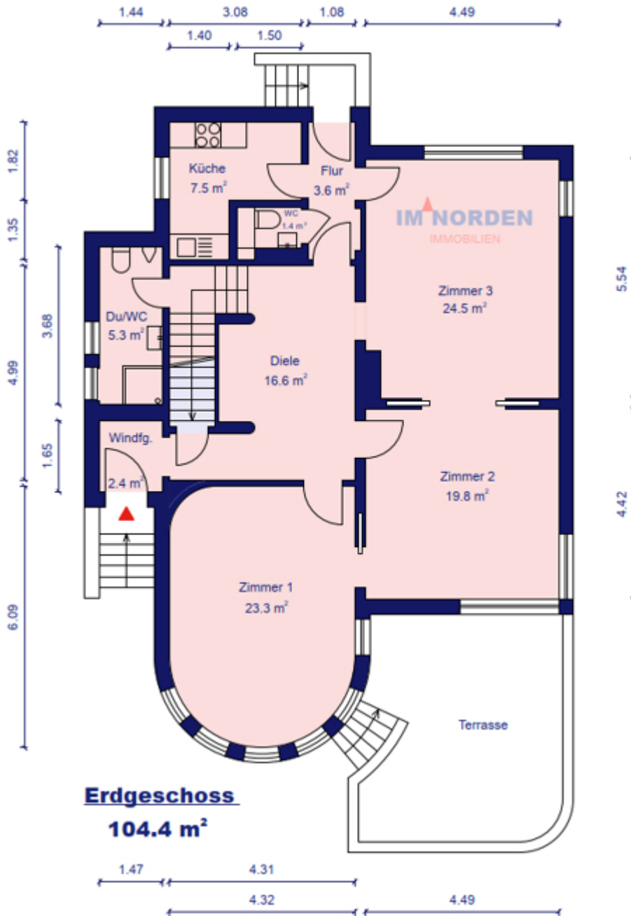
Grundriss Erdgeschoss
